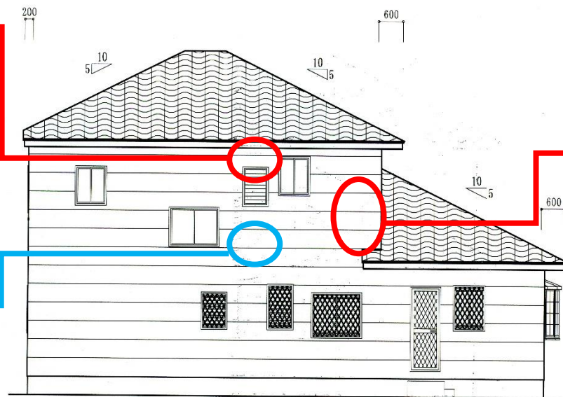
南侧 立面图 S: 1/100
